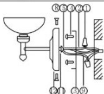
Imagen 3 Lámpara de pared
