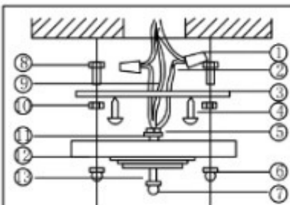
Imagen 1 Lámpara de techo
